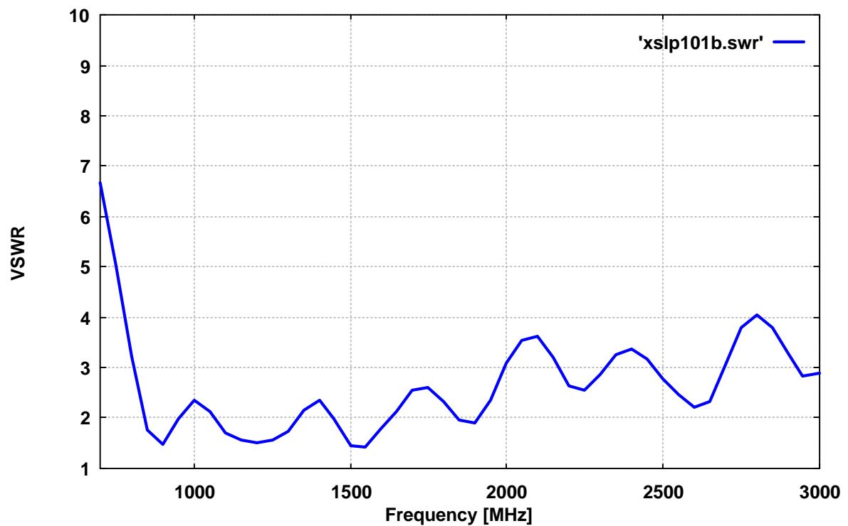
VSWR an der N-Buchse "B" XSLP 9142
