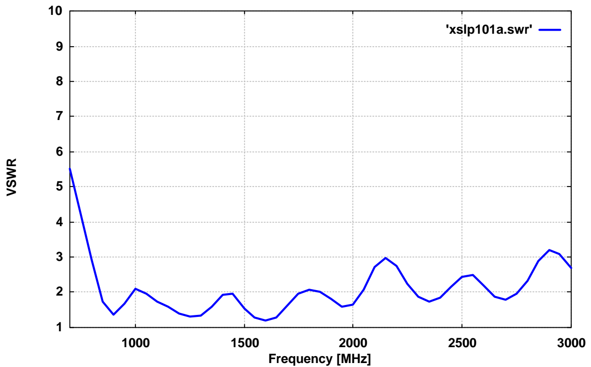
VSWR an der N-Buchse "A" XSLP 9142
